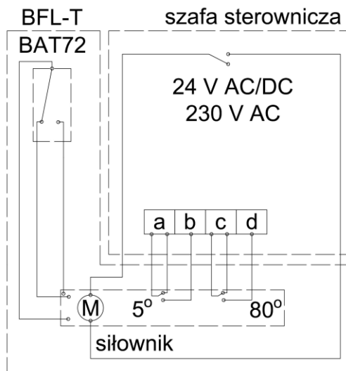
Rysunek 9. Schemat ideowy instalacji elektrycznej dla kłap w wariancie ER z siłownikiem BFL-T
