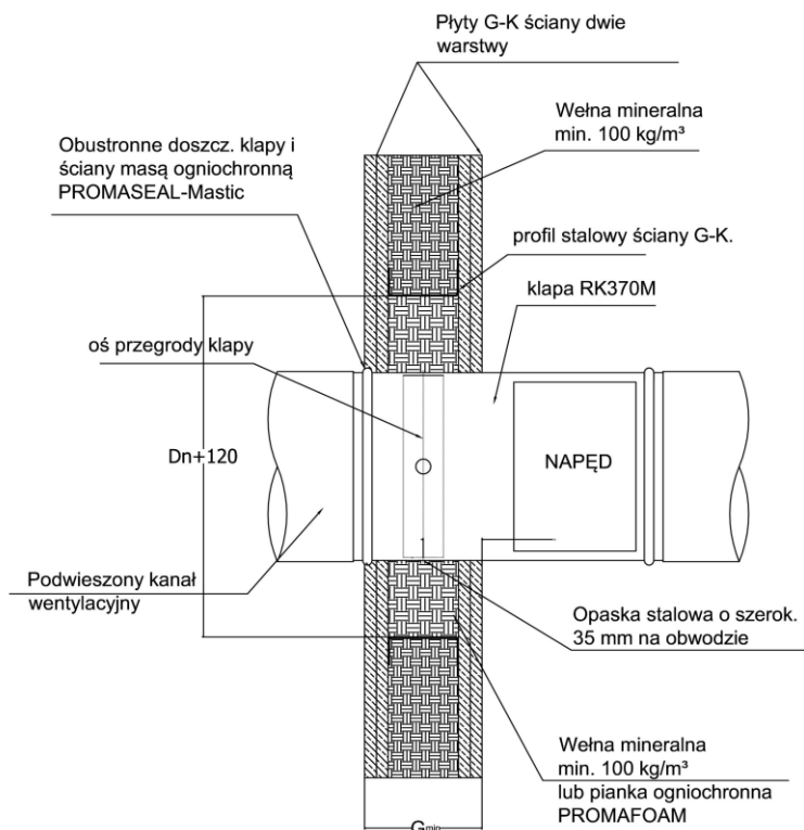
Rysunek 7. Przykład montażu klapy RK370M w ścianach typu lekkiego z płyt gipsowo-kartonowych (zabudowa klap z równoczesnym montażem przewodów wentylacyjnych)
