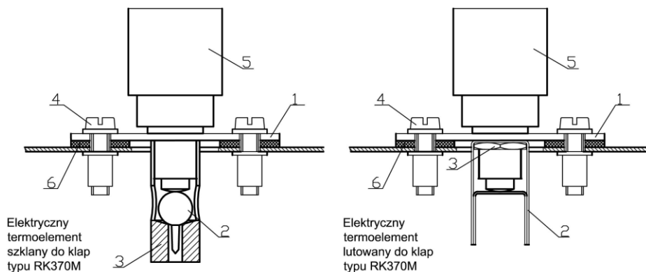
Rysunek 13. Opis i budowa termoelementów klapy RK370M MR
