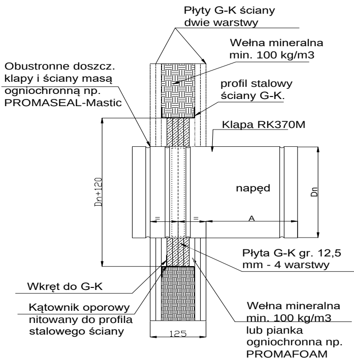
Rysunek 6. Przykład montażu klap RK370M w ścianach typu lekkiego z płyt gipsowo-kartonowych (zabudowa klap przed montażem przewodów wentylacyjnych)
