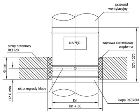
Rysunek 5. Przykład montażu kłapy RK370M w stropach betonowych – napęd nad stropem
