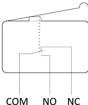
Rysunek 11. Schemat połączeń mikroprzełącznika klapy RK370M
